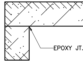
BUTT EDGE WITH APRON
